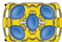
ADD6 Arreglo para bandejas 254 x 368 mm y platos Ø 191 y 254 mm.
